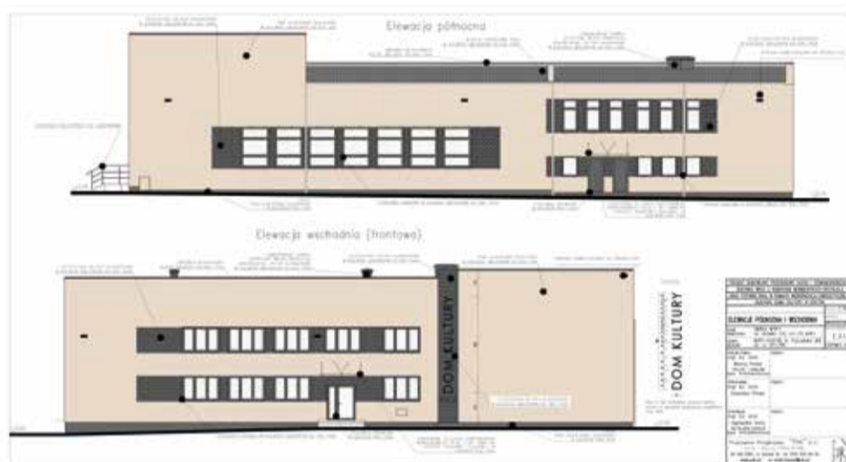
Projekt elewacji północnej i wschodniej (frontowe)
